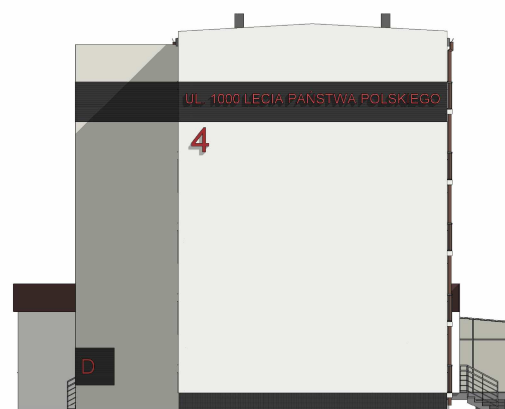
ELEWACJA PÓŁNOCNA
